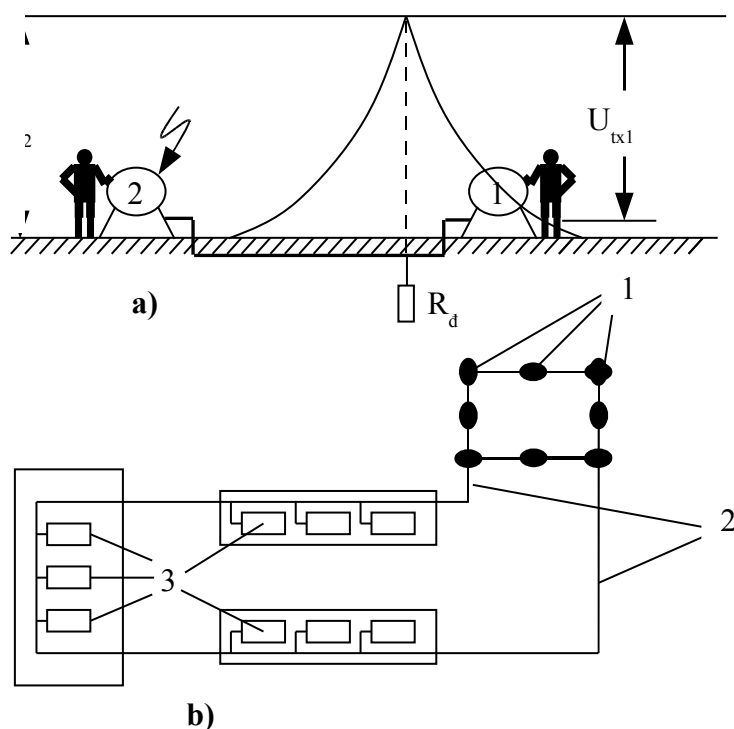
Hình 4.2: Nối đất tập trung
