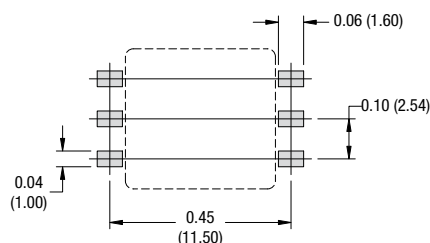
6 Pin SM
