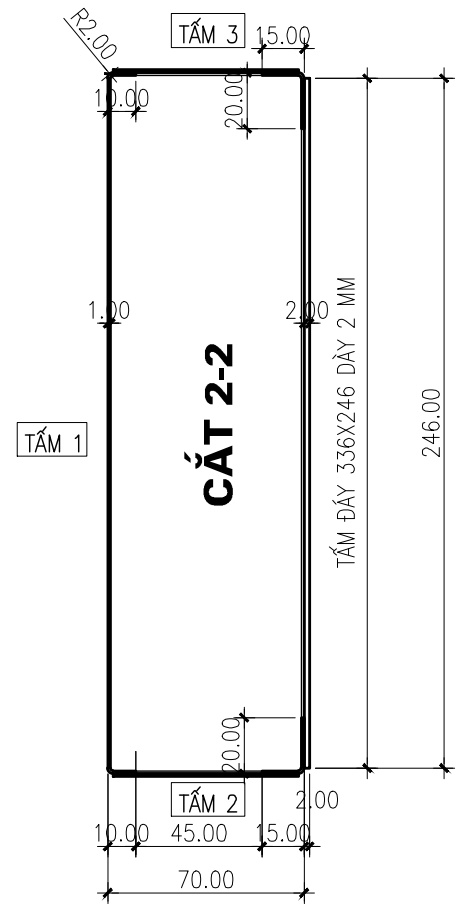
MẶT BẰNG
